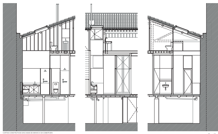
CORTES CONSTRUCTIVO DAS CASAS DE BANHO E DA COBERTURA
