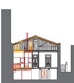
ALTERAÇÕES - C1 - CORTE TRANSVERSAL
