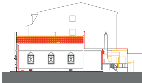
ALTERAÇÕES - ALÇADO VESTE
